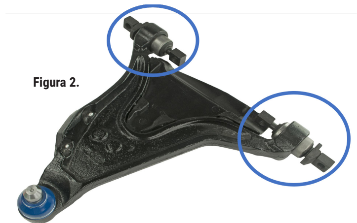
Figura 2. Tipo 2: comúnmente se denomina "Estilo de 4 pernos", ya que se requieren 4 pernos del buje al bastidor.
