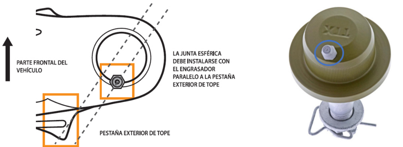
Figura 1. Para asegurar el espacio libre adecuado entre los componentes, la junta esférica debe instalarse con el conector de grasa en paralelo a la pestaña exterior de tope inferior
