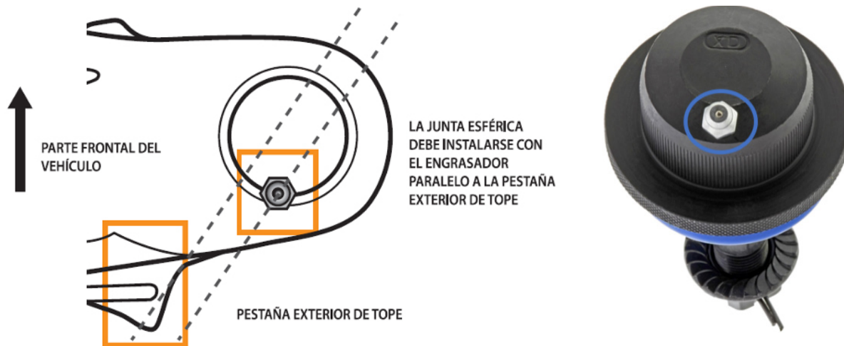
Figura 1. Para asegurar el espacio libre adecuado entre los componentes, la junta esférica debe instalarse con el conector de grasa en paralelo a la pestaña exterior de tope inferior
