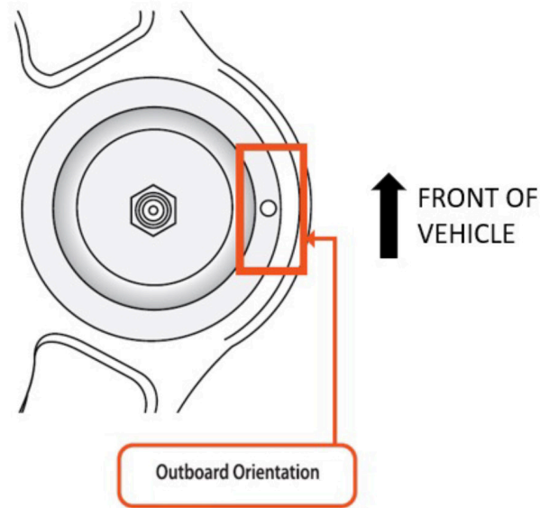
Figura 3. Orientación correcta de la instalación de la junta esférica cuando se acopla con el brazo de control delantero superior de acero forjado. Observe la posición de la marca de referencia (rectángulo anaranjado).
