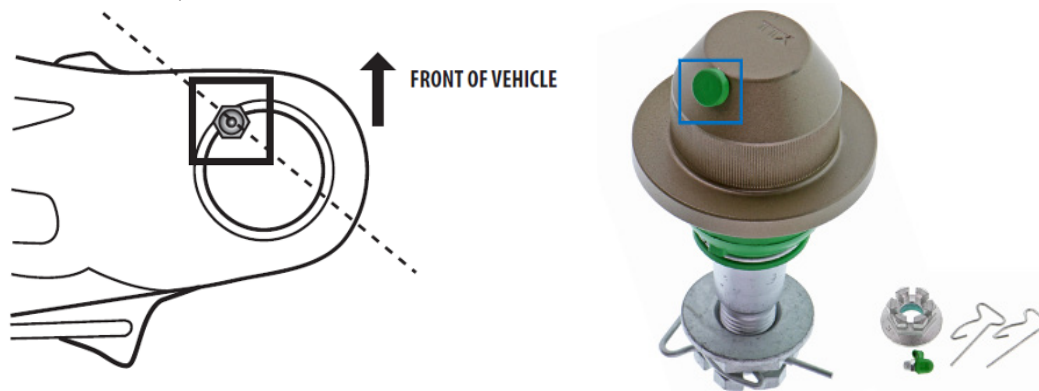
Figura 1. Para asegurar el espacio libre adecuado entre los componentes, la junta esférica debe instalarse con el conector de grasa a aproximadamente 45° hacia el centro del vehículo.
