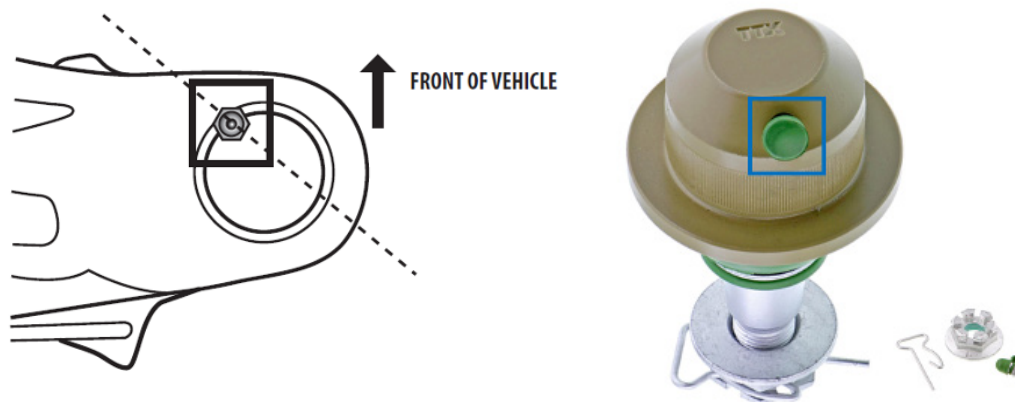
Figura 1. Para asegurar el espacio libre adecuado entre los componentes, la junta esférica debe instalarse con el conector de grasa a aproximadamente 45° hacia el centro del vehículo.
