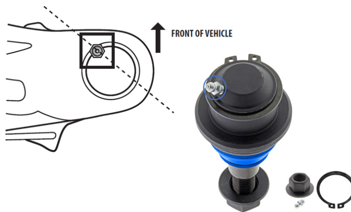
Figura 1. Para asegurar el espacio libre adecuado entre los componentes, la junta esférica debe instalarse con el conector de grasa a aproximadamente 45° hacia el centro del vehículo.
