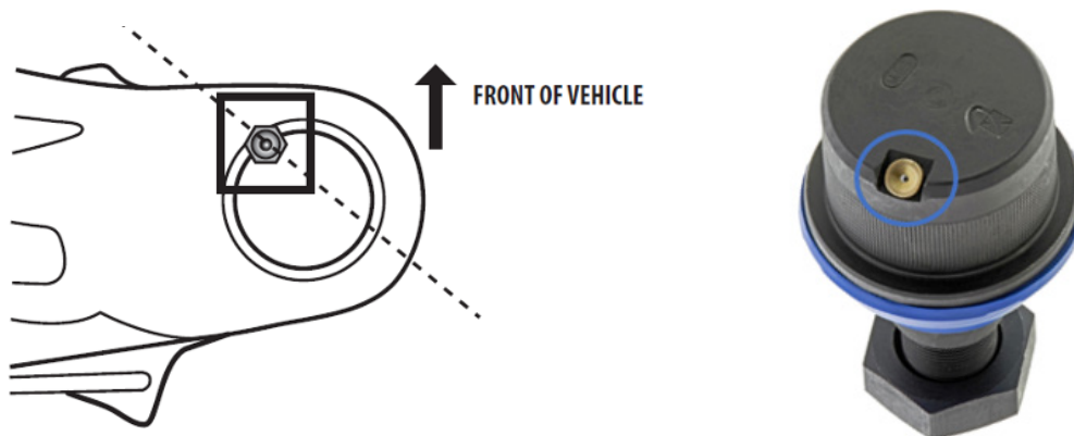
Figura 1. Para asegurar el espacio libre adecuado entre los componentes, la junta esférica debe instalarse con el conector de grasa a aproximadamente 45° hacia el centro del vehículo.
