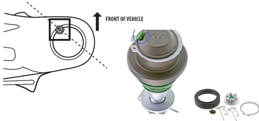
Figura 1. Para asegurar el espacio libre adecuado entre los componentes, la junta esférica debe instalarse con el conector de grasa a aproximadamente 45° hacia el centro del vehículo.
