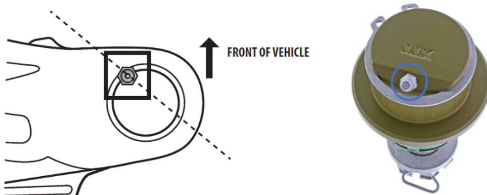
Figura 1. Para asegurar una mejora en la facilidad del servicio de lubricación, la junta esférica debe instalarse con el conector de grasa a aproximadamente 45° hacia el centro del vehículo.
