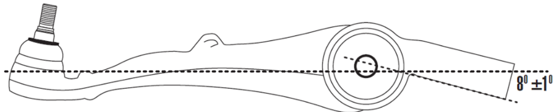
Figura 2. La orientación correcta se logra al alinear la línea de centro del brazo de control con el borde inferior del soporte dentro de 8^\circ (\pm 1^\circ) .
