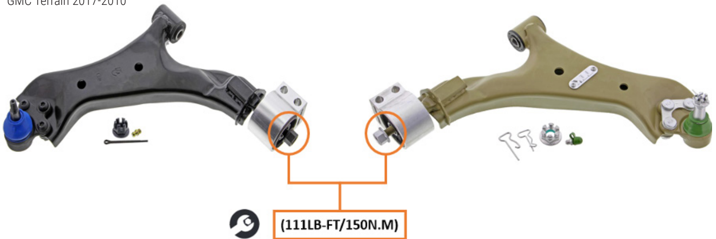
Figura 1. La tuerca del soporte del buje (encerrada en un círculo arriba) debe apretarse correctamente después de colocar el brazo de control en el vehículo
