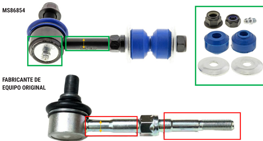
Figura 1. La barra de conexión estabilizadora trasera MS86854 Supreme de Mevotech con hardware de reemplazo y bujes, barra de acoplamiento de mayor diámetro y rodamientos sinterizados autolubricantes (arriba) vs fabricante de equipo original (abajo)
