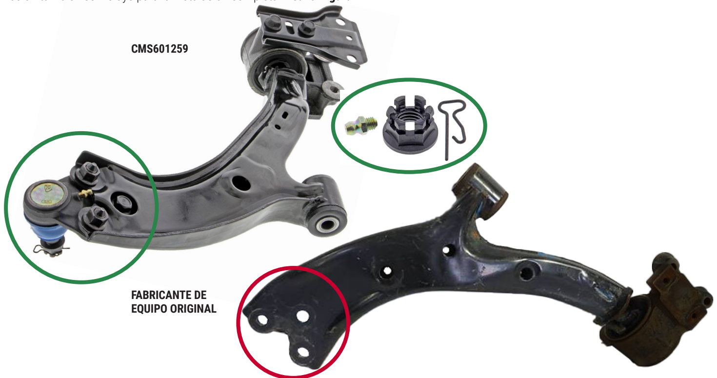
Figura 1. Conjunto del brazo de control delantero inferior hacia adelante Supreme de Mevotech CMS601259 con junta esférica preinstalada y hardware (arriba) vs brazo de control básico estilo fabricante de equipo original (abajo)
