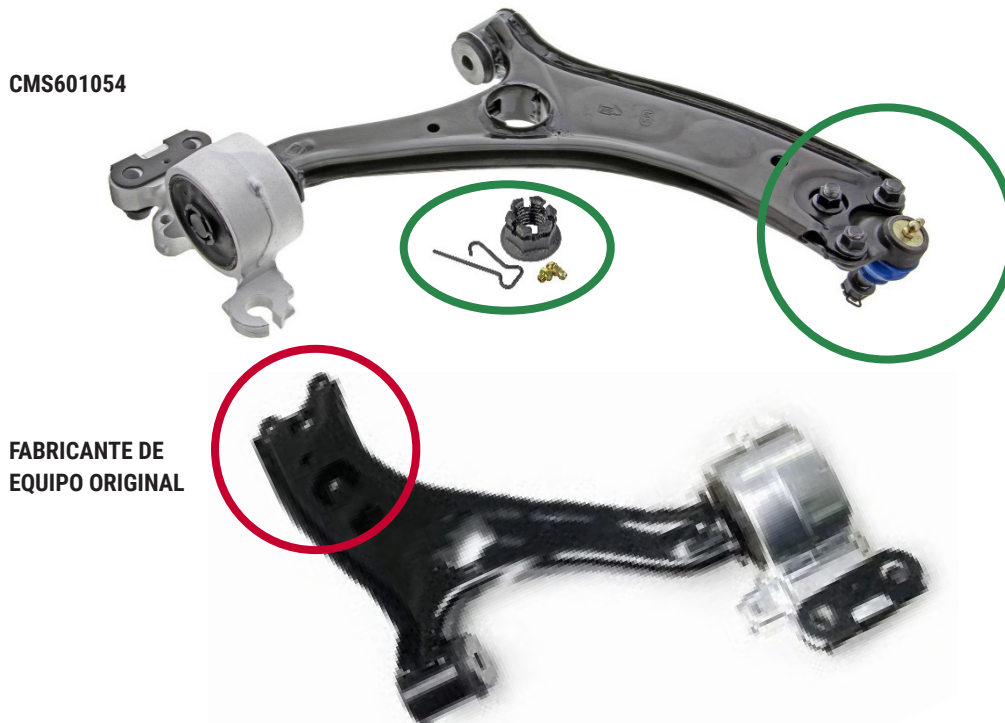
Figura 1. El conjunto de brazo de control delantero inferior hacia adelante CMS601054 de Supreme de Mevotech con una junta esférica de ingeniería integrada y con hardware (arriba) vs brazo de control de fabricante de equipo original básico (abajo)
