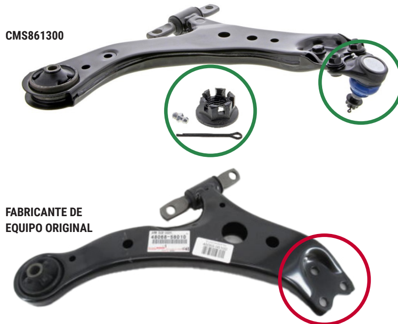
Figura 1. El conjunto de brazo de control delantero inferior hacia adelante CMS861300 con una junta esférica diseñada integrada y con hardware (arriba) vs brazo de control de Fabricante de equipo original básico (abajo)
