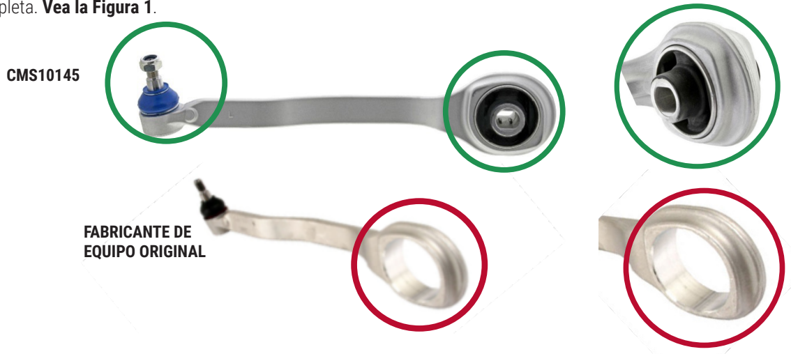
Figura 1. Brazo de control Supreme de Mevotech CMS10145 con buje preinstalado y hardware (arriba) vs brazo de control básico estilo fabricante de equipo original (abajo)
