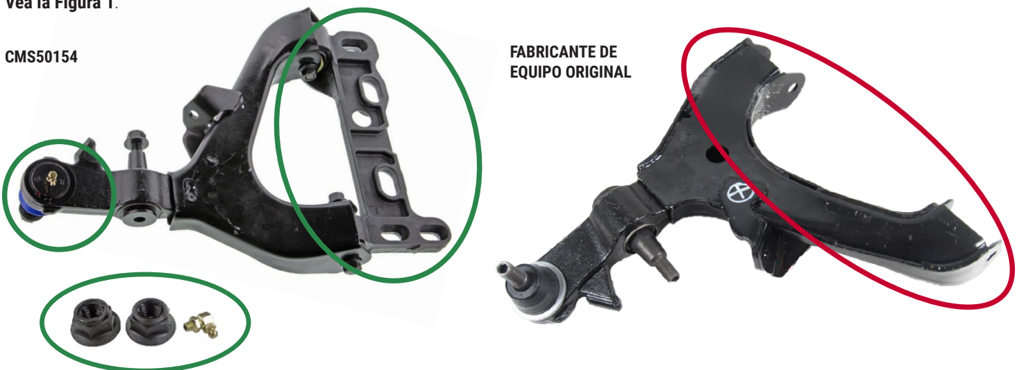
Figura 1. Brazo de control delantero inferior Supreme de Mevotech CMS50154 con soporte de montaje preensamblado, junta esférica sinterizada, engrasable, autolubrificante y hardware (izquierda) vs brazo de control de fabricante de equipo original (derecha)
