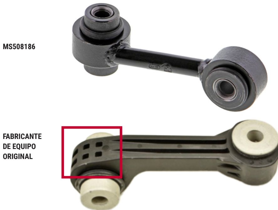
Figura 1. La barra de conexión estabilizadora Supreme de Mevotech MS508186 con cuerpo con recubrimiento anticorrosivo de acero (arriba) vs cuerpo plástico con cavidades del fabricante de equipo original (abajo)
