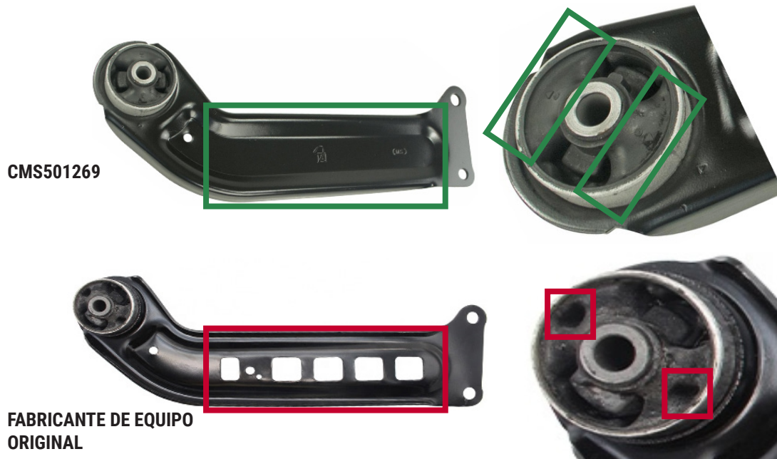
Figura 1. El brazo de arrastre trasero Supreme de Mevotech CMS501269 con perfil estampado mejorado con un cuerpo relleno y huecos de buje (arriba) vs diseño de fabricante de equipo original (abajo)
