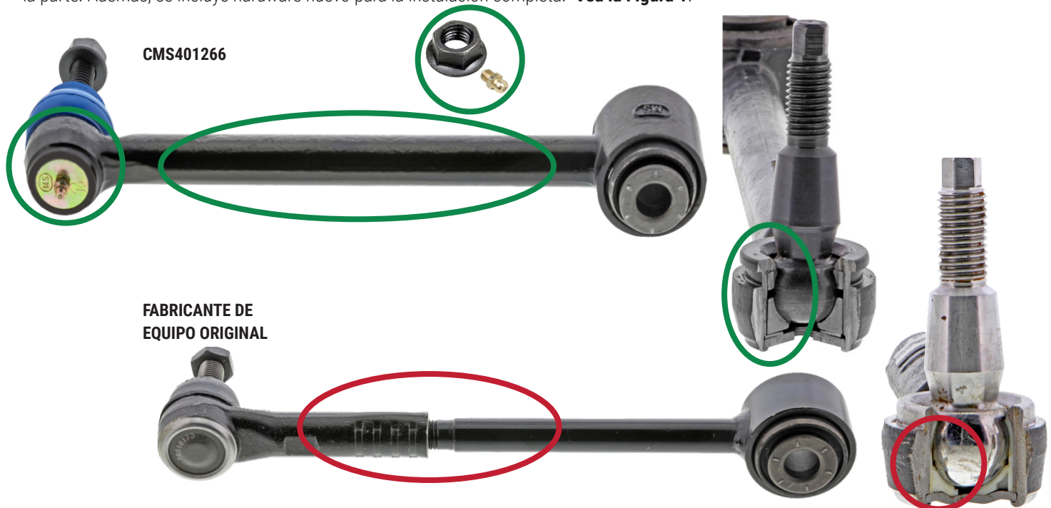
Figura 1. Barra de conexión lateral Supreme de Mevotech con rodamientos de metal superior e inferior sinterizados engrasables autolubricantes y forjado sólido de una pieza (arriba) vs diseño de dos piezas de brazo de control y rodamiento de plástico de fabricante de equipo original (abajo)
