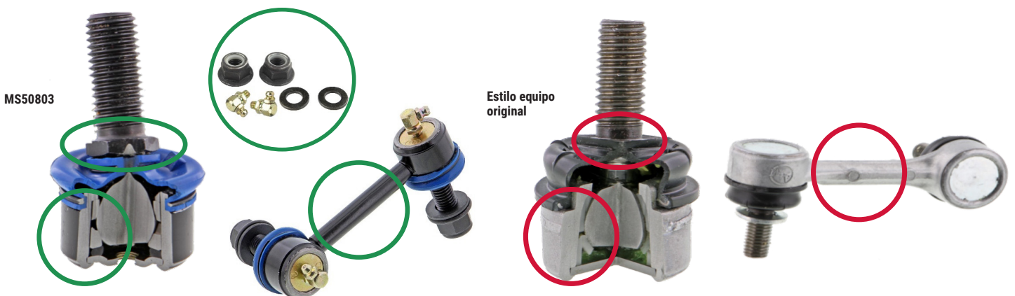
Figura 1. Barra de conexión estabilizadora Supreme de Mevotech MS50803 con diseño de acero sólido, con rodamientos de metal sinterizado superior e inferior engrasables autolubricantes, superficie plana mejorada para llave para facilitar la instalación y hardware incluido (izquierda) vs rodamiento de plástico sellado de fabricante de equipo original, superficie plana para llave reducida y diseño de aluminio ligero (derecha)
