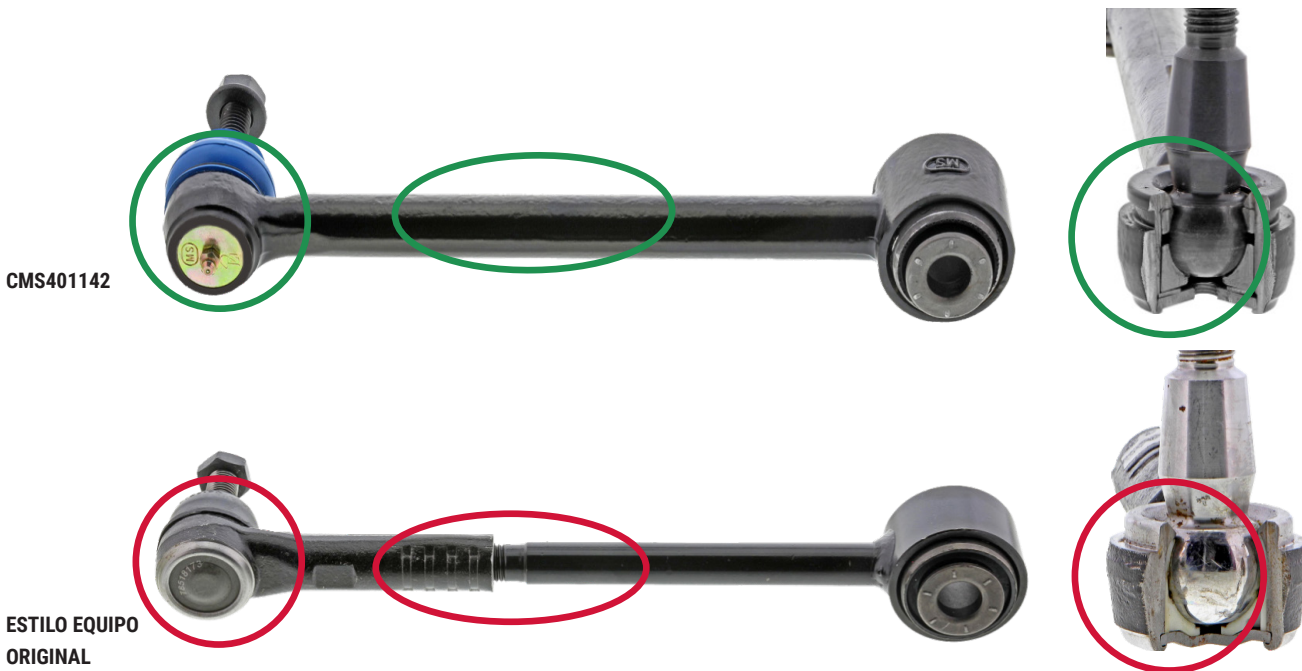
Figura 1. Brazo de control Supreme de Mevotech con rodamientos superior e inferior de metal sinterizado autolubricantes y engrasables y forjado mejorado de una pieza sólida (arriba) vs diseño de dos piezas de brazo de control estilo equipo original y rodamiento de plástico (abajo)
