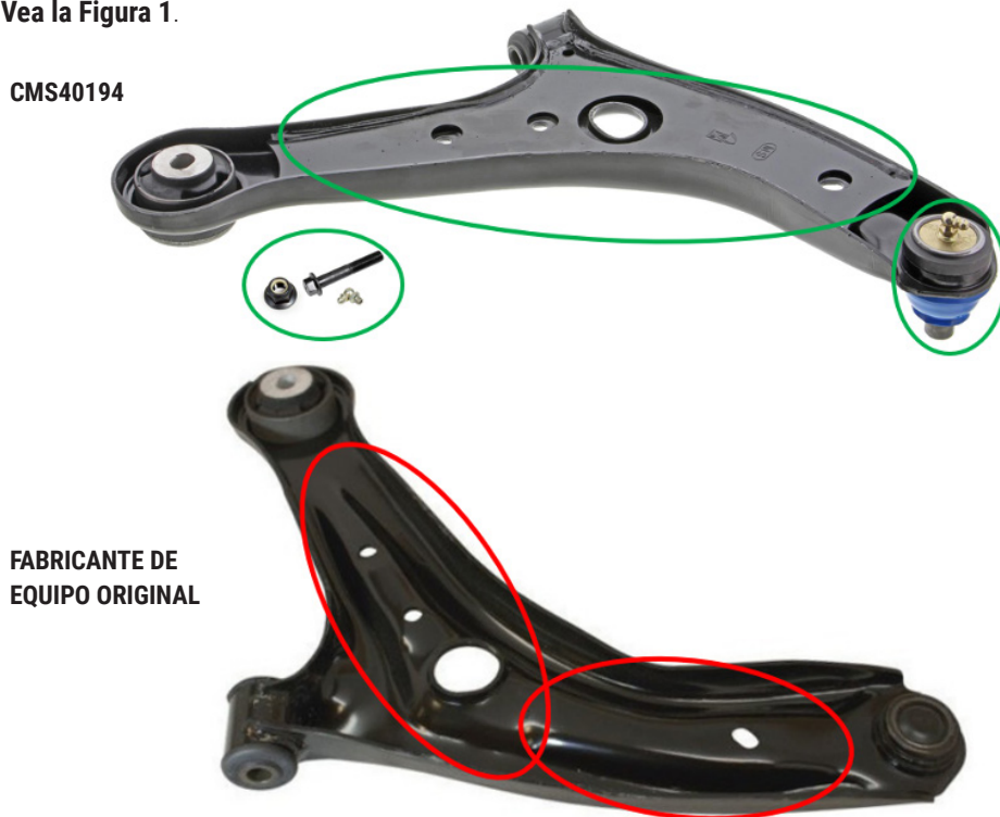
Figura 1. Brazo de control Supreme de Mevotech CMS40194 con perfil estampado mejorado, placa de refuerzo, junta esférica de rodamiento sinterizado engrasable autolubricado y hardware incluido (arriba) vs diseño de fabricante de equipo original (abajo)
