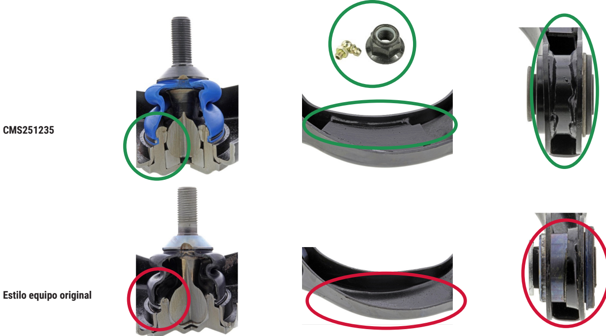
Figura 1. Brazo de control Supreme de Mevotech CMS251235 con perfil de acero estampado mejorado y rodamientos de metal sinterizado superior e inferior autolubricantes engrasables, refuerzo adicional del bastidor y bujes, y hardware incluido (arriba) vs diseño de fabricante de equipo original y junta esférica que no puede recibir servicio (abajo)
