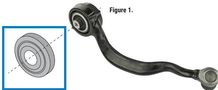
Figure 1. Les bras de suspension avant inférieurs avant Mevotech Supreme CMS101483 et CMS101484 sont conçus pour loger le bouclier de bague d'origine (mis en évidence dans l'encadré bleu à droite).
