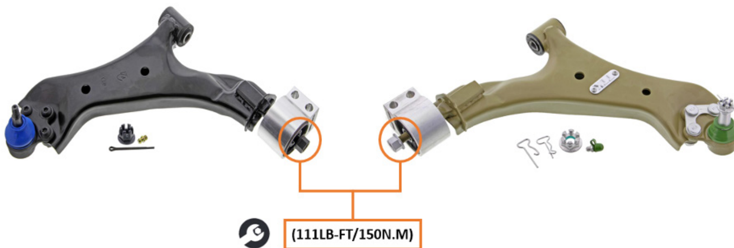
Figure 1. L'écrou de support de bague (encerclé plus haut) doit être serré correctement après l'installation du bras de suspension sur le véhicule.
