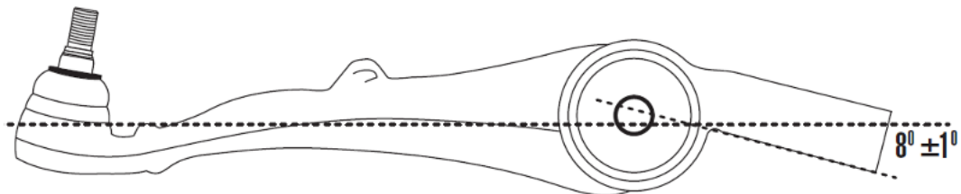
Figure 2. L'orientation adéquate est obtenue lorsque la ligne centrale du bras de suspension et le bord inférieur du support sont alignés à 8^\circ (\pm 1^\circ) .
