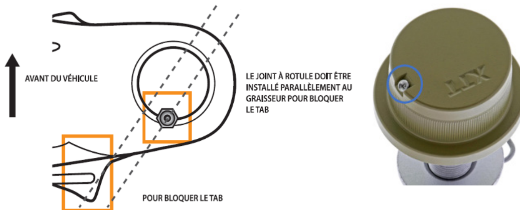
Figure 1. Pour assurer un dégagement adéquat entre les composants, le joint à rotule doit être installé parallèlement à la languette d'arrêt inférieure.
