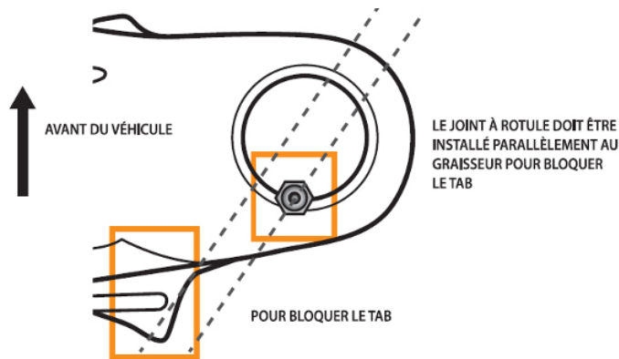
Figure 1. Pour assurer un dégagement adéquat entre les composants et permettre une accessibilité lors des prochains entretiens de lubrification, le joint à rotule doit être installé parallèlement à la languette d'arrêt du bras de suspension inférieur avant.
