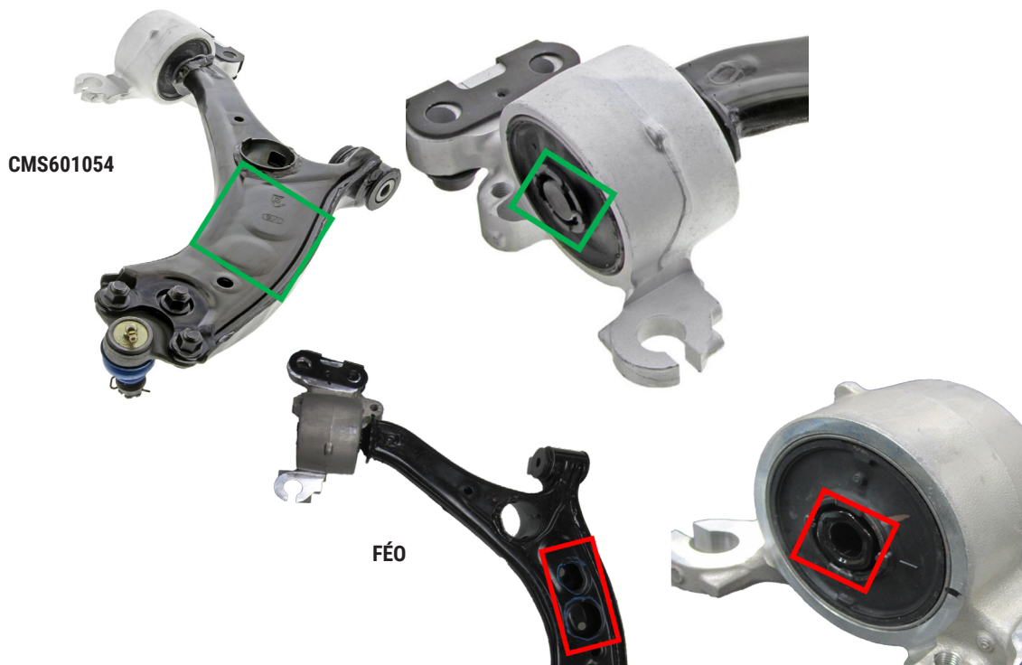
Figure 1. Bras de suspension inférieur avant Mevotech Supreme CMS601054 avec profil d'estampage amélioré présentant des cavités remplies et un arbre de bague plein (haut) comparativement à la conception d'origine (bas)
