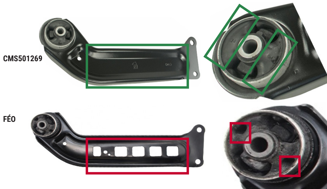
Figure 1. Bras oscillants arrière Mevotech Supreme CMS501269 avec profil d'estampage amélioré et cavités du corps et des bagues remplies (haut) comparativement à la conception d'origine (bas)
