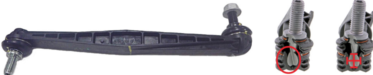
Figure 1. Pièce Mevotech Supreme MS258128 présentant une conception en acier massif avec paliers supérieurs et inférieurs en métal fritté autolubrifiants et graissables et une plus grande surface de contact entre le pivot de rotule et le palier ainsi que la quincaillerie incluse (haut) par rapport au corps en plastique de la pièce d'origine, au logement en plastique scellé et à la surface de contact réduite du pivot à rotule (bas)
