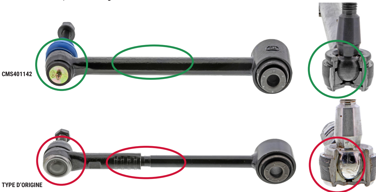
Figure 1. Bras de suspension Mevotech Supreme avec paliers supérieur et inférieur en métal fritté autolubrifiants et graissables et pièce forgée massive améliorée (en haut) comparativement au bras de suspension d'origine en deux pièces et aux paliers en plastique (en bas)
