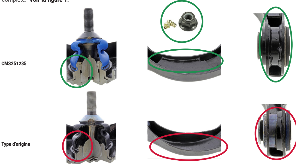
Figure 1. Bras de suspension CMS251235 Supreme de Mevotech fabriqué selon un profil d'acier estampé amélioré comprenant des paliers en métal fritté supérieurs et inférieurs autolubrifiants et graissables, un renfort supplémentaire au châssis et à la bague ainsi que du matériel inclus (en haut) comparativement au modèle du joint à rotule non utilisable du FEO (en bas).
