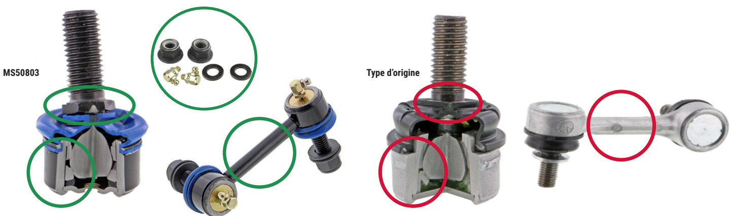
Figure 1. Embout de barre stabilisatrice avant Mevotech Supreme MS50803 en acier massif, avec paliers supérieurs et inférieurs en métal fritté graissables et autolubrifiants, plat de clé amélioré pour une installation plus facile et matériel inclus (à gauche) par rapport aux paliers en plastique scellés d'origine, plat de clé réduit et conception légère en aluminium (droite).
