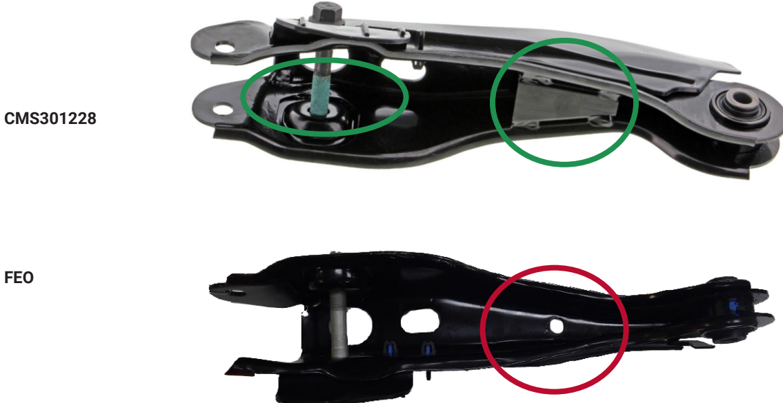
Figure 1. Bras de suspension Mevotech Supreme CMS301228 avec profil d'estampage amélioré et plaque de renforcement, et quincaillerie revêtue d'un adhésif frein-filet (haut) par rapport à la conception d'origine (bas).
