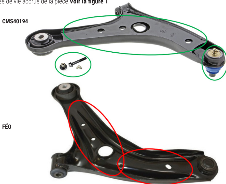
Figure 1. Bras de suspension Mevotech Supreme CMS40194 avec profil d'estampage amélioré et plaque de renforcement, un palier en métal fritté autolubrifiant à raccord de graissage et la quincaillerie incluse (haut) par rapport à la conception d'origine (bas).
