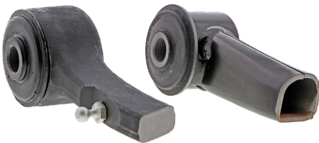
Figure 1 : Conception forgée solide Mevotech (à gauche) vs conception vide en acier estampé d'origine (à droite)
