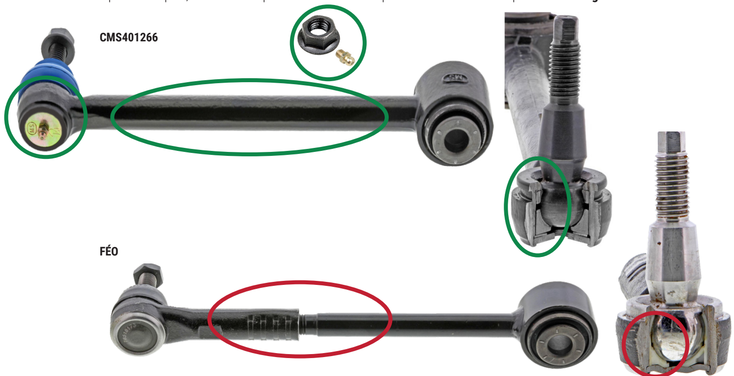
Figure 1. Bras latéral Mevotech Supreme à conception en acier avec paliers supérieurs et inférieurs en métal fritté autolubrifiants à raccord de graissage et pivot de rotule monopièce amélioré (haut), comparativement à la conception en deux pièces du bras de suspension d'origine et au palier en plastique (bas)
