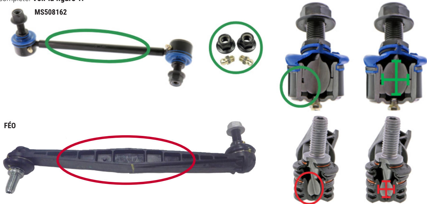
Figure 1. Pièce Mevotech Supreme MS508162 présentant une conception en acier massif avec paliers supérieurs et inférieurs en métal fritté autolubrifiants et graissables et une plus grande surface de contact entre le pivot de rotule et le palier ainsi que la quincaillerie incluse (haut) par rapport au corps en plastique de la pièce d'origine, au logement en plastique scellé et à la surface de contact réduite du pivot à rotule (bas)
