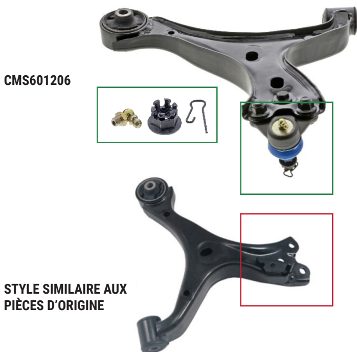
Figure 1. Ensemble de bras de suspension inférieur avant Mevotech Supreme CMS601206 avec joint à rotule modifié préinstallé et quincaillerie (haut) par rapport au bras de suspension nu de style similaire aux pièces d'origine (bas)
