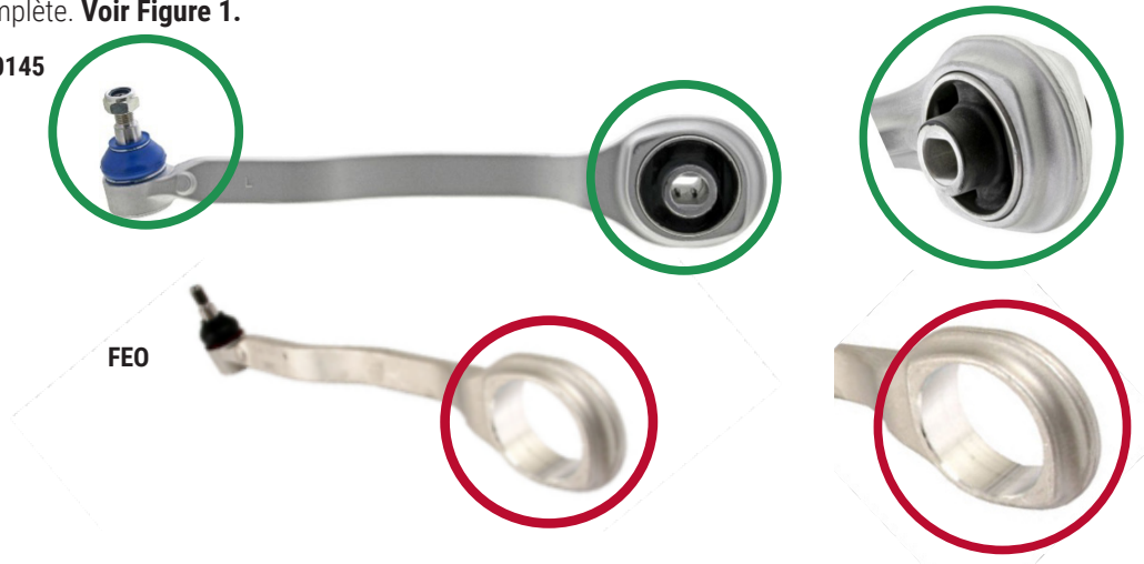
Figure 1. Bras de suspension Mevotech Supreme CMS10145 avec bague prémontée et quincaillerie de fixation (haut) comparativement au bras de suspension d'origine nu (bas).
