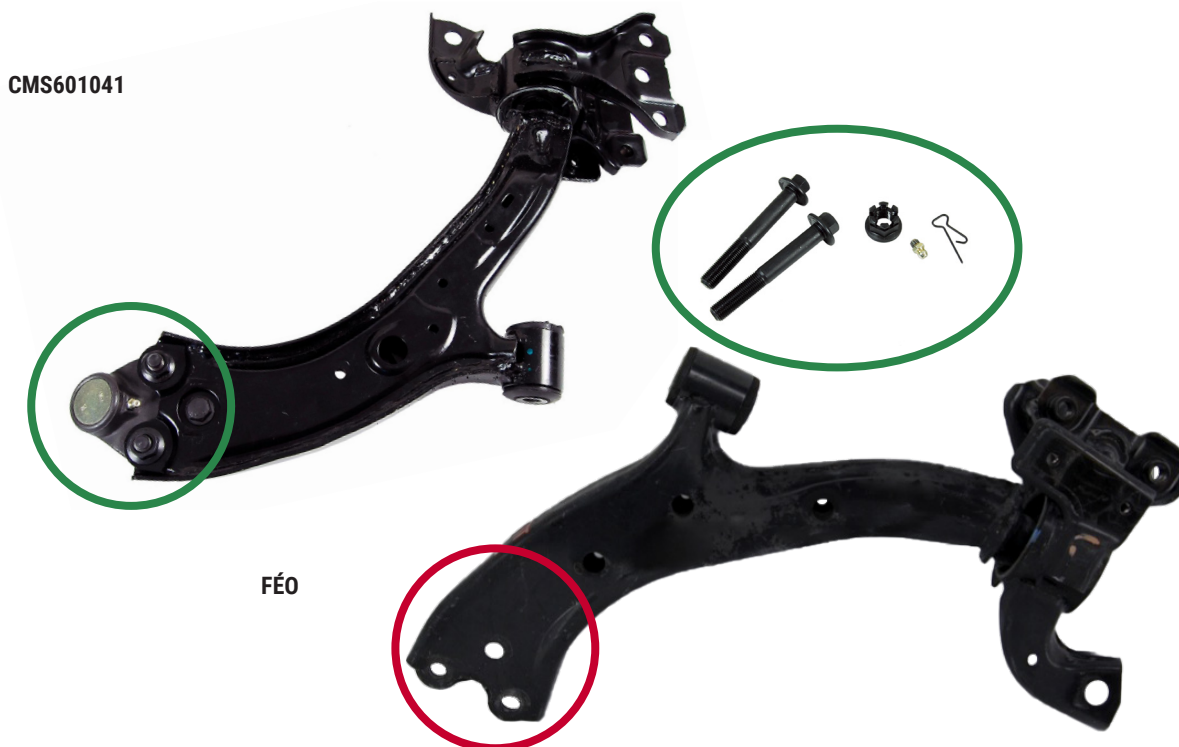
Figure 1. Bras de suspension avant inférieur avant Mevotech Supreme CMS601041 avec joint à rotule prémonté et quincaillerie (haut) vs bras de suspension d'origine nu (bas)
