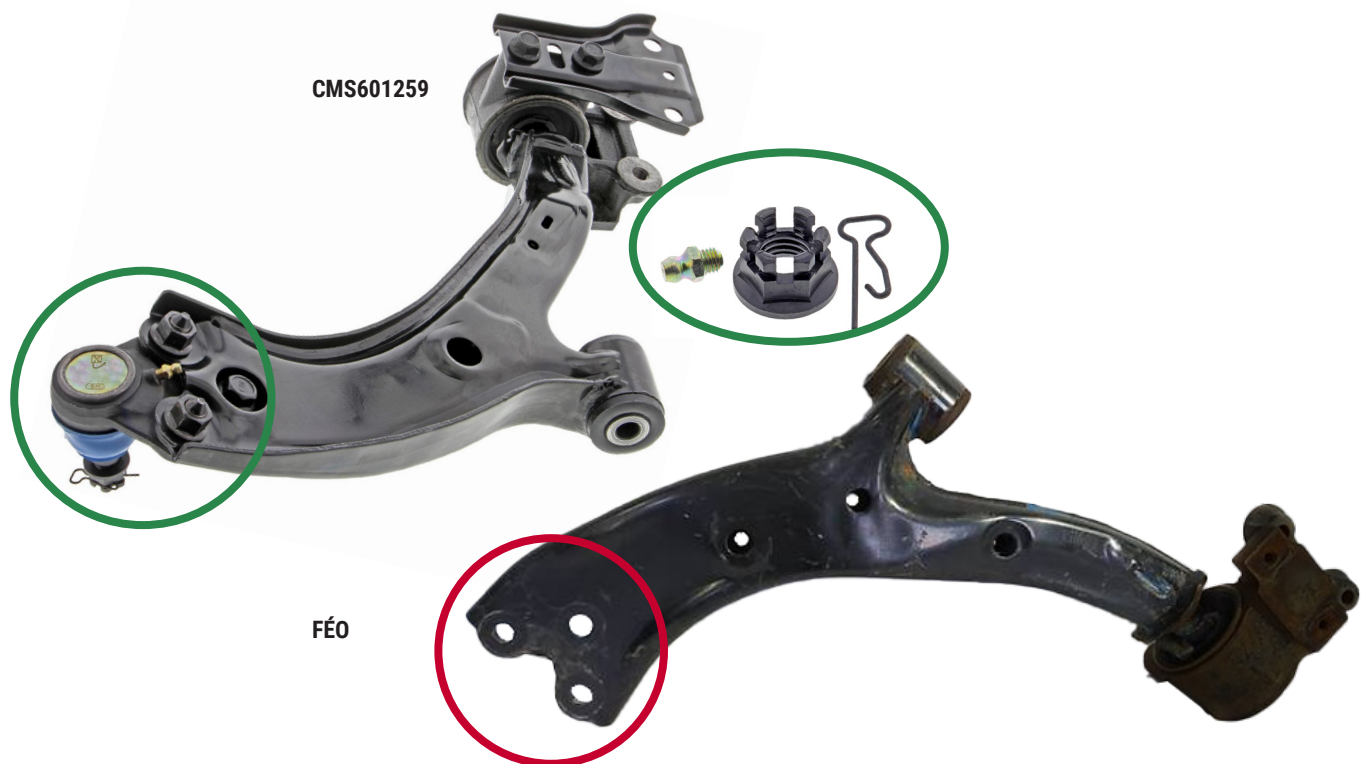
Figure 1. Bras de suspension avant inférieur avant Mevotech Supreme CMS601259 avec joint à rotule prémonté et quincaillerie (haut) vs bras de suspension d'origine nu (bas)
