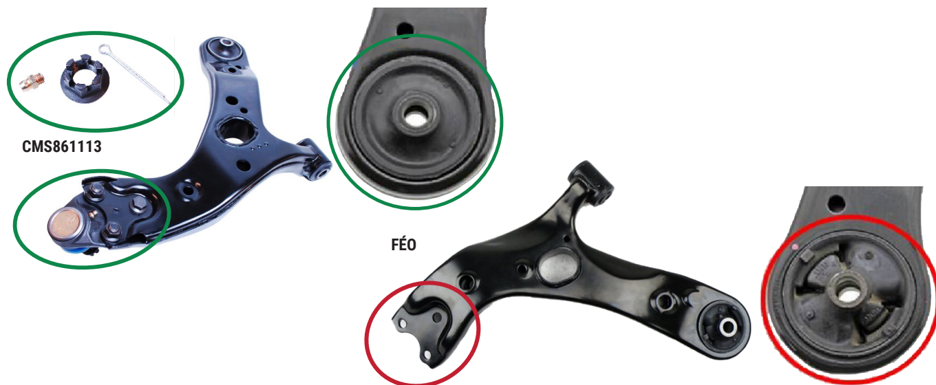
Figure 1. Bras de suspension inférieur avant Mevotech Supreme CMS861113 avec joint à rotule prémonté et quincaillerie (haut) comparativement au bras de suspension d'origine nu (bas)
