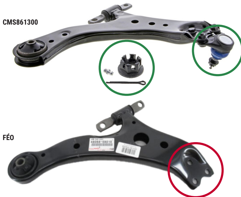
Figure 1. Ensemble de bras de suspension inférieur avant vers l'avant Mevotech Supreme CMS861300 avec joint à rotule modifié prémonté et quincaillerie (haut) comparativement au bras de suspension d'origine nu (bas)
