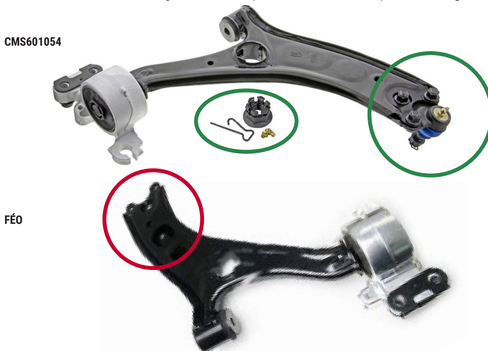
Figure 1. Ensemble de bras de suspension inférieur avant vers l'avant Mevotech Supreme CMS601054 avec joint à rotule modifié prémonté et quincaillerie (haut) comparativement au bras de suspension d'origine nu (bas)
