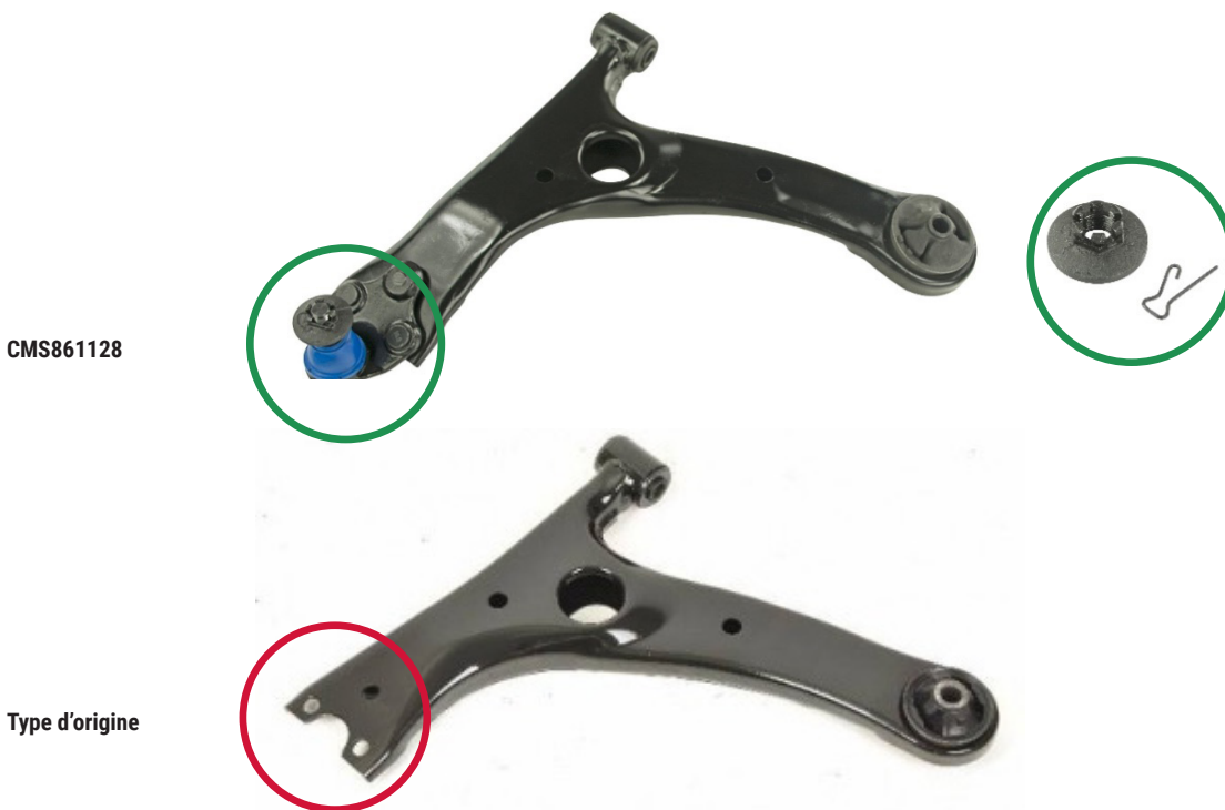
Figure 1. Bras de suspension Mevotech Supreme avec joint à rotule prémonté et matériel inclus (en haut) comparativement au bras de suspension d'origine nu (en bas)
