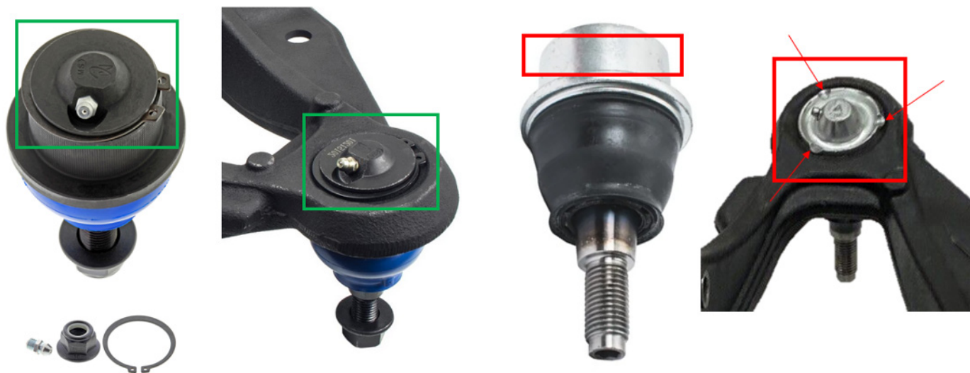
Figure 1. Le joint à rotule inférieur avant Mevotech Supreme MS50553 peut être fixé au bras de suspension facilement grâce au circlip (gauche) comparativement à la méthode de fixation ou de sertissage de la conception d'origine (droite)
